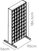
60 Door Locker Stand Fixed
